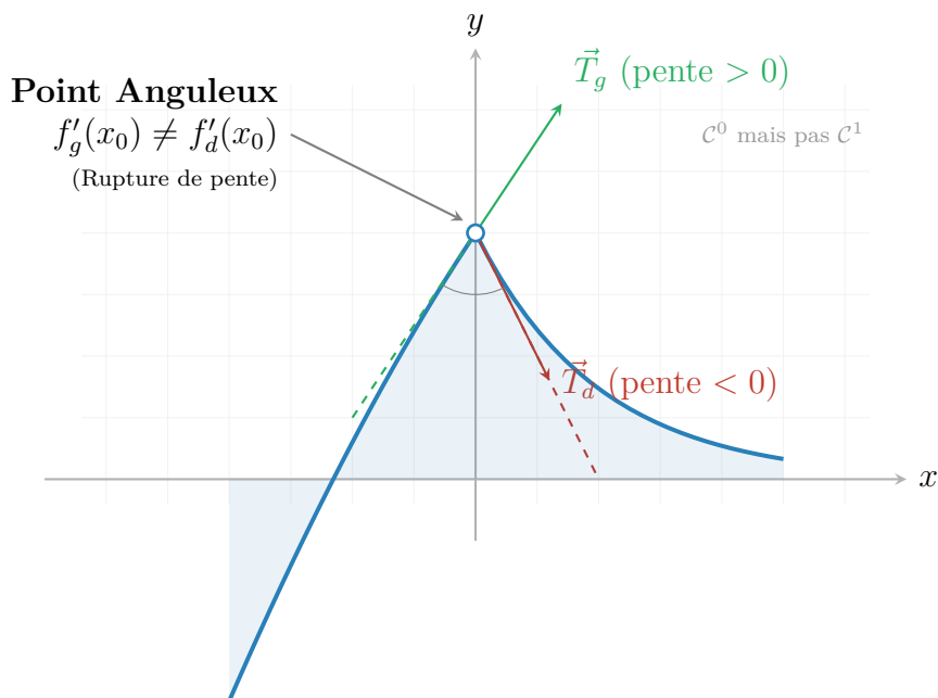
Figure 1.1 – Représentation graphique d'une fonction continue non dérivable en x = 0 . Le changement brusque de la pente (de positive à gauche à négative à droite) crée un point anguleux caractéristique.
