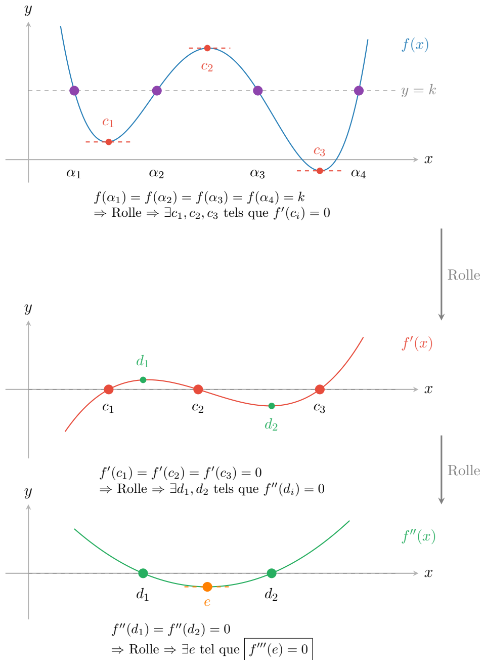
Figure 2.1 – Illustration de l'exercice : Application successive du théorème de Rolle. Si f prend la même valeur en n + 1 = 4 points, alors f' s'annule en 3 points, puis f'' s'annule en 2 points, et finalement f^{(3)} s'annule en au moins 1 point.
